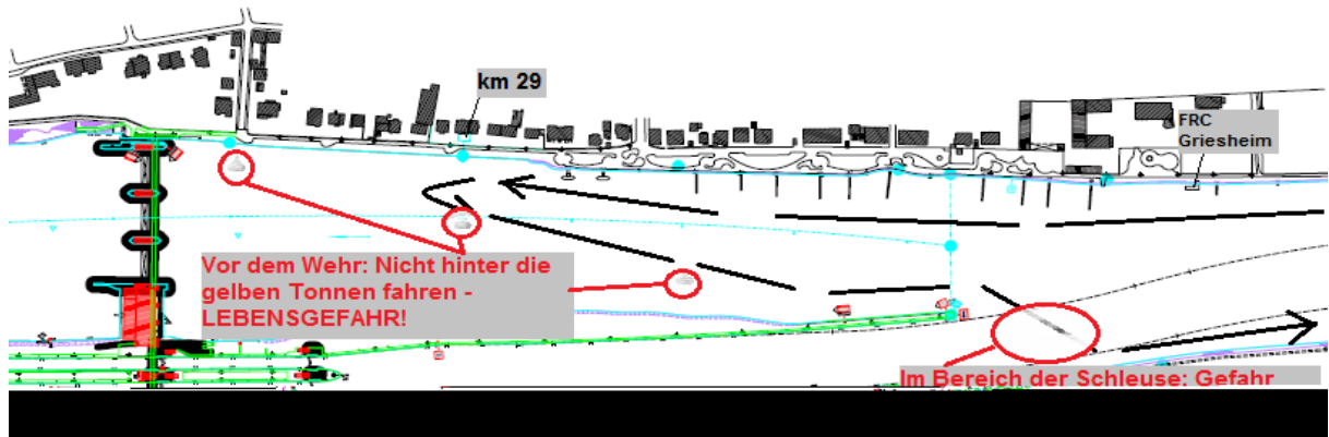
ABBILDUNG 3: Schleuse Griesheim
